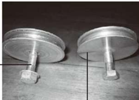
巻取器側滑車軸 ネット巻きでワイヤーを 巻く分摩耗が激しい
